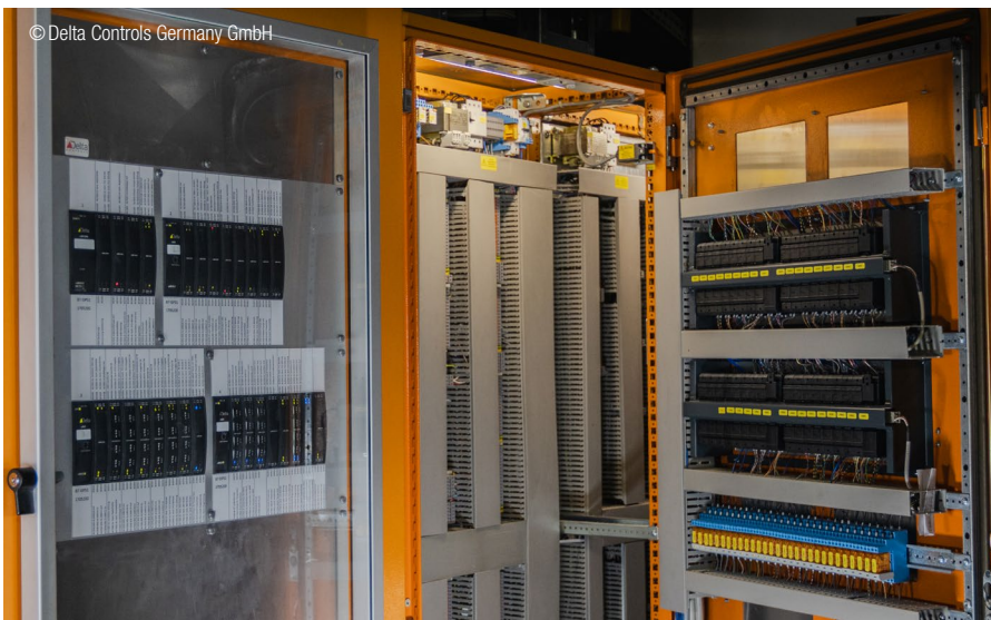
Gebäudeautomatenschaltschrank im Keller der Gebäude am Potsdamer Platz. Building automation control cabinet in the basement of the buildings at Potsdamer Platz.
